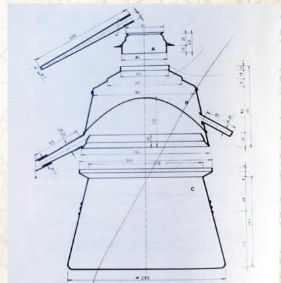
Bakır imbiğin kesit şeması. A: Kapak, B: Soğutucu, C: Kazan.
